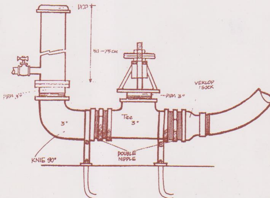
Gambar 2 : Bentuk Pompa Hydran
