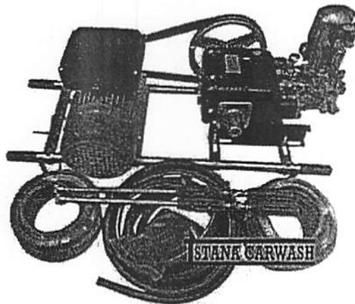
Gambar 7. Alat/Mesin yang akan diberikan ke mitra
